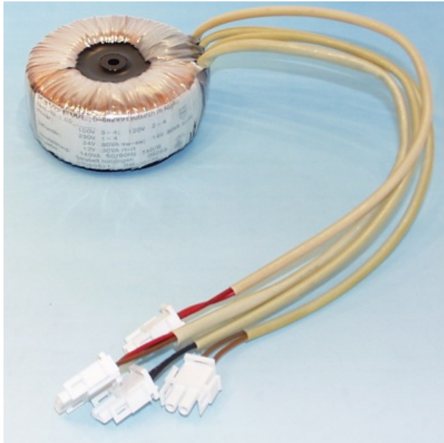
Ringkerntransformator mit Mittellochverguss
